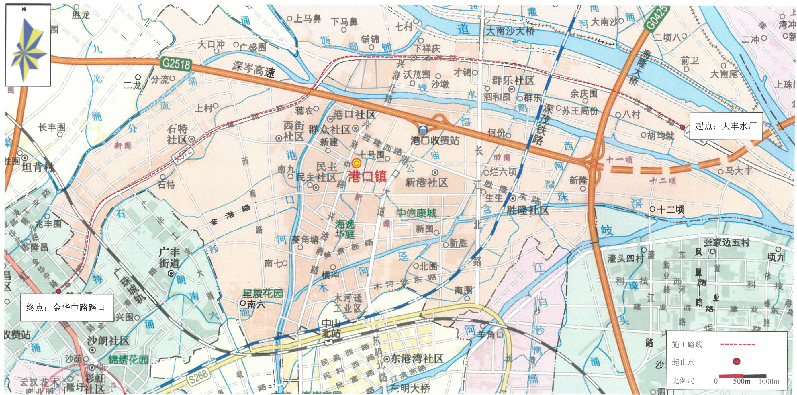
图1 沙港路供水管网互联互通保障工程施工路线图
